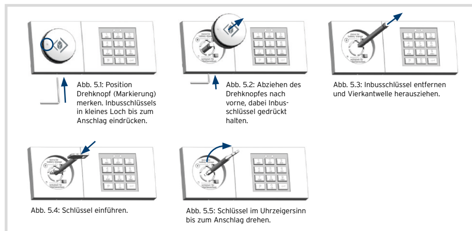
Abbildung 5: Schlüsselöffnung
