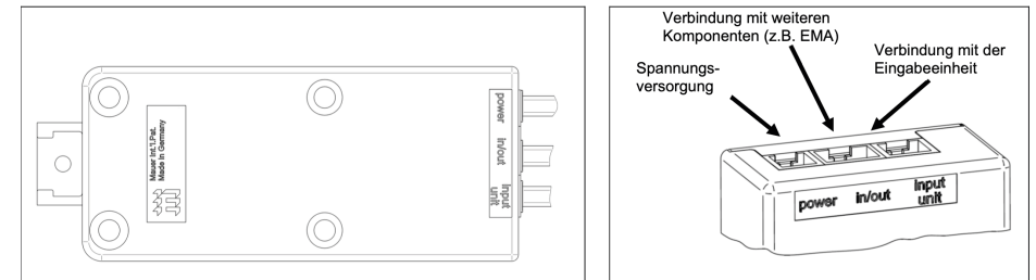
Abbildung 3: Schlossgehäuse
