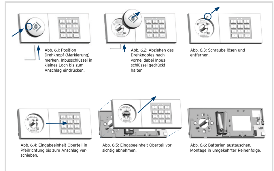
Abbildung 6: Batterietausch
