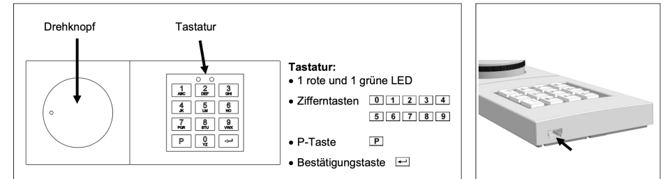
Abbildung 1: Eingabeeinheit
